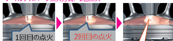
火炎核の成長が速く、燃焼が良い
